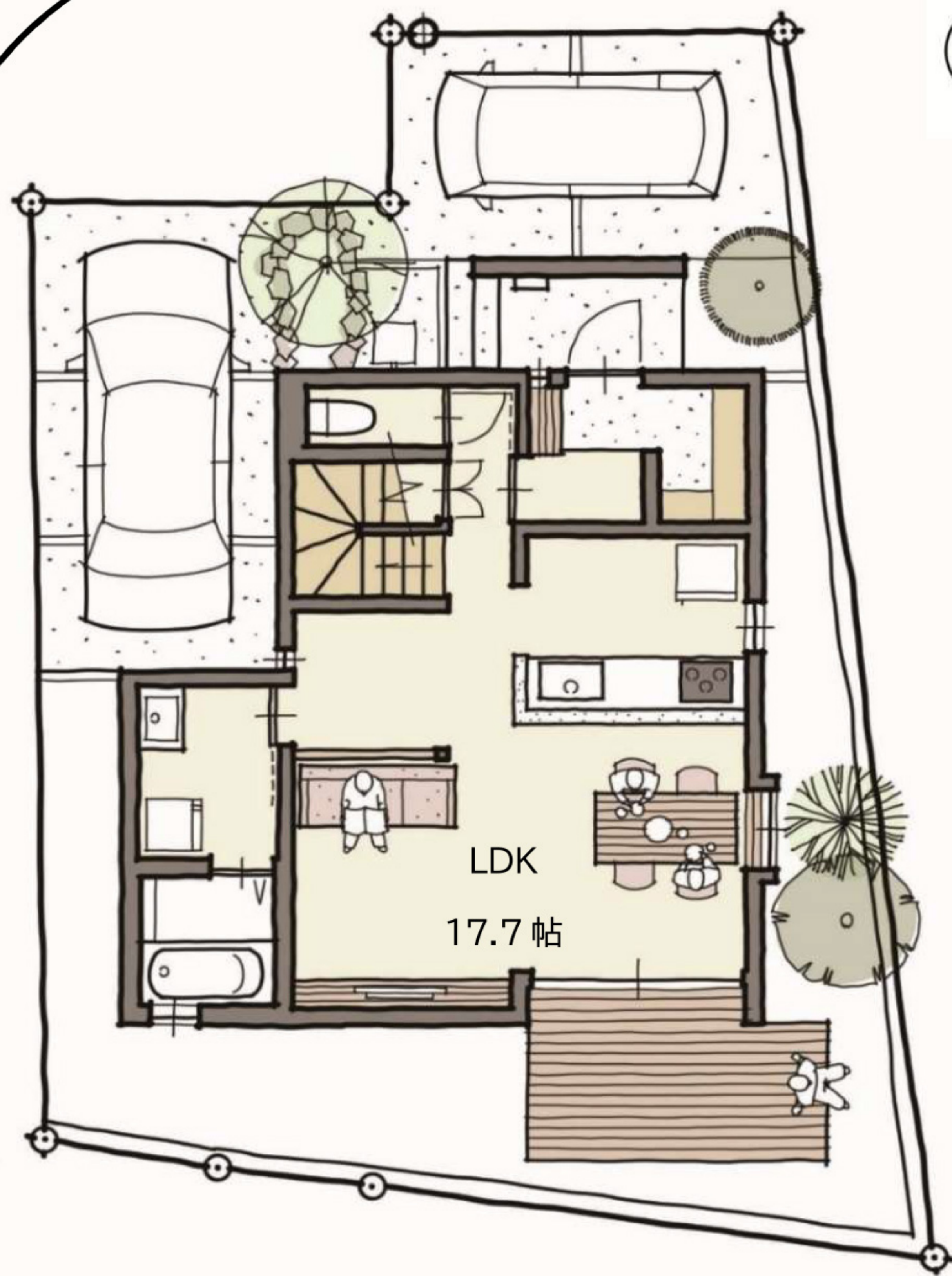
配置図・1階平面図
