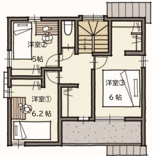
2階平面図
