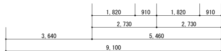
● 1階 平面図 S:1/100
